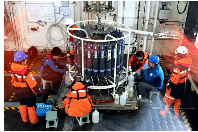
2025年8月19日，科考队员在采集CTD（温盐深剖面仪）带回的水样品。（新华社记者 刘诗平 摄）
